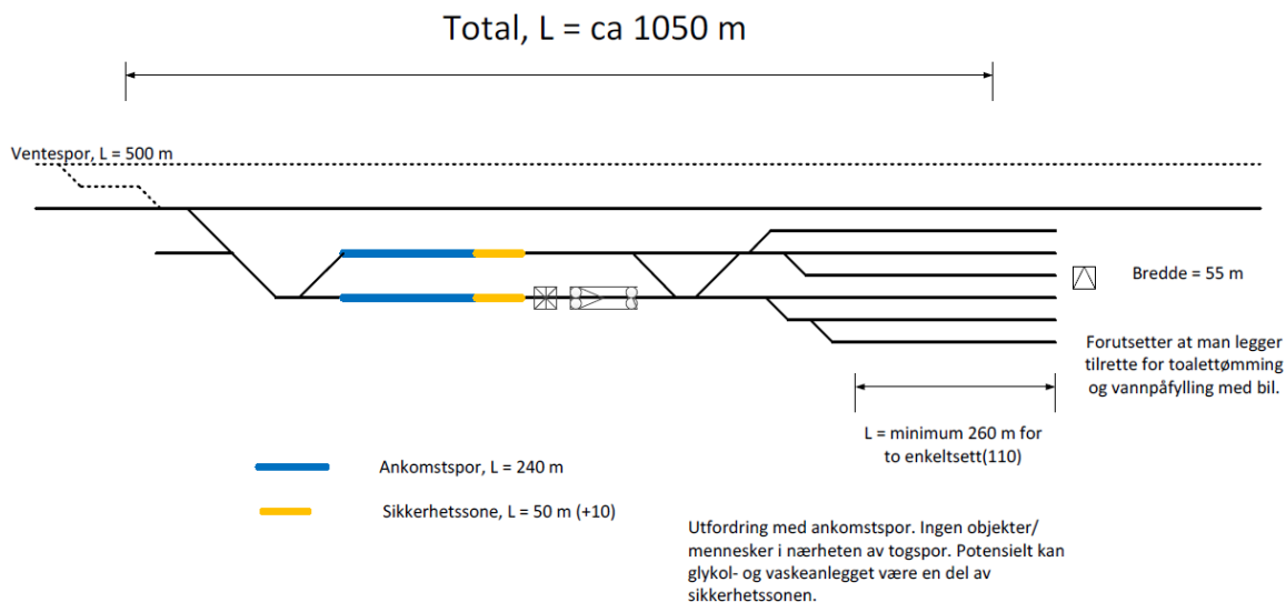
Fig 2.3 Anbefalt utforming av driftsbanegård med 8-16 plasser hvor det er behov for togspor (ankomst/avgangsspor) inne på driftsbanegården
