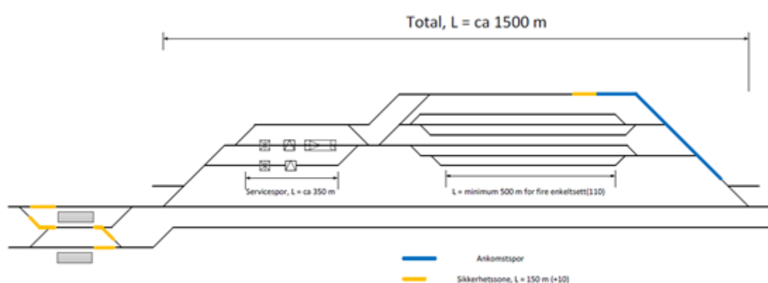
Fig. 2.6 Anbefalt utforming av en større driftsbanegård enn 16-20 plasser
