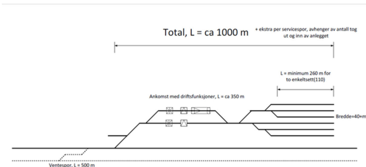
Fig. 2.4 Anbefalt utforming av driftsbanegård med 8-16 plasser, tilknyttet ventespør eller stasjon
