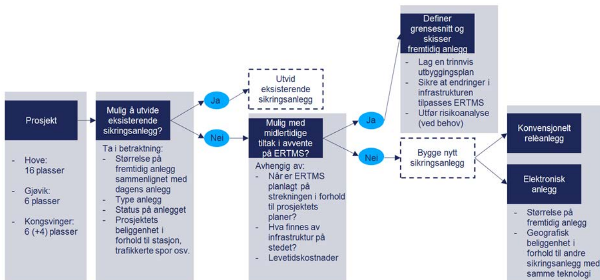
Fig. 3.1 Metodikk for vurdering av sikringsanlegg på nye driftsbanegårder. Fra «Notat – Signal og sikringsanlegg for hensettingsområder», Plan og teknikk 25.08.17
