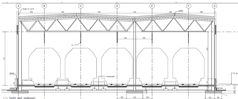
Fig. 4.3 Eksempel på overbygget hensetting
