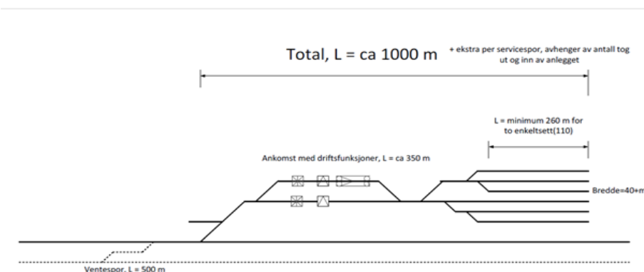
Fig. 2.4 Anbefalt utforming av driftsbanegård med 8-16 plasser, tilknyttet ventespør eller stasjon
