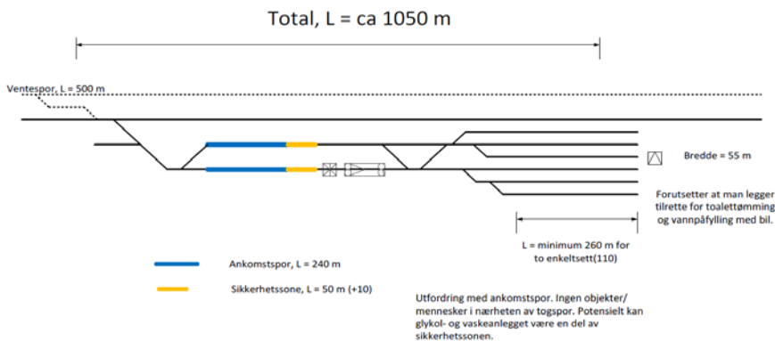
Fig 2.3 Anbefalt utforming av driftsbanegård med 8-16 plasser hvor det er behov for togspor (ankomst/avgangsspor) inne på driftsbanegården
