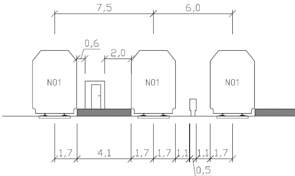
Figur 5.1. Eksempel på plassering av servicekiosk og togvarmeposter
