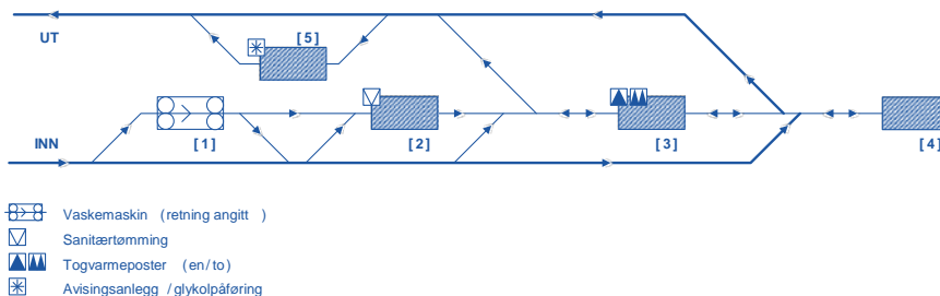
Figur 2.2: Prinsipiell fremstilling (eksempel) av et optimalt hensettingsanlegg. (1) utvendig vask, (2) innvendig vask/sanitærtømming, (3) hensettingsspor, (4) verksted, (5) avisinganlegg. Avisinganlegget kan også plasseres like etter utvendig vask og innvendig vask skje på hensettingsspor – også sanitærtømming hvis den skjer med bil. Kilde: Strategisk rammeverk for stoppesteder, Dokumentasjonsrapport, utarbeidet av Rambøll for Jernbaneverket
