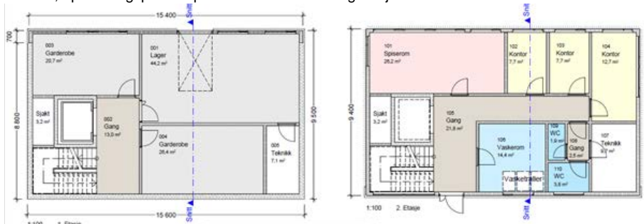
Fig. 4.4 Plantegning av servicebygg (eksempel)
