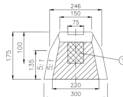
A-A Armeringsfritt tverrsnitt
