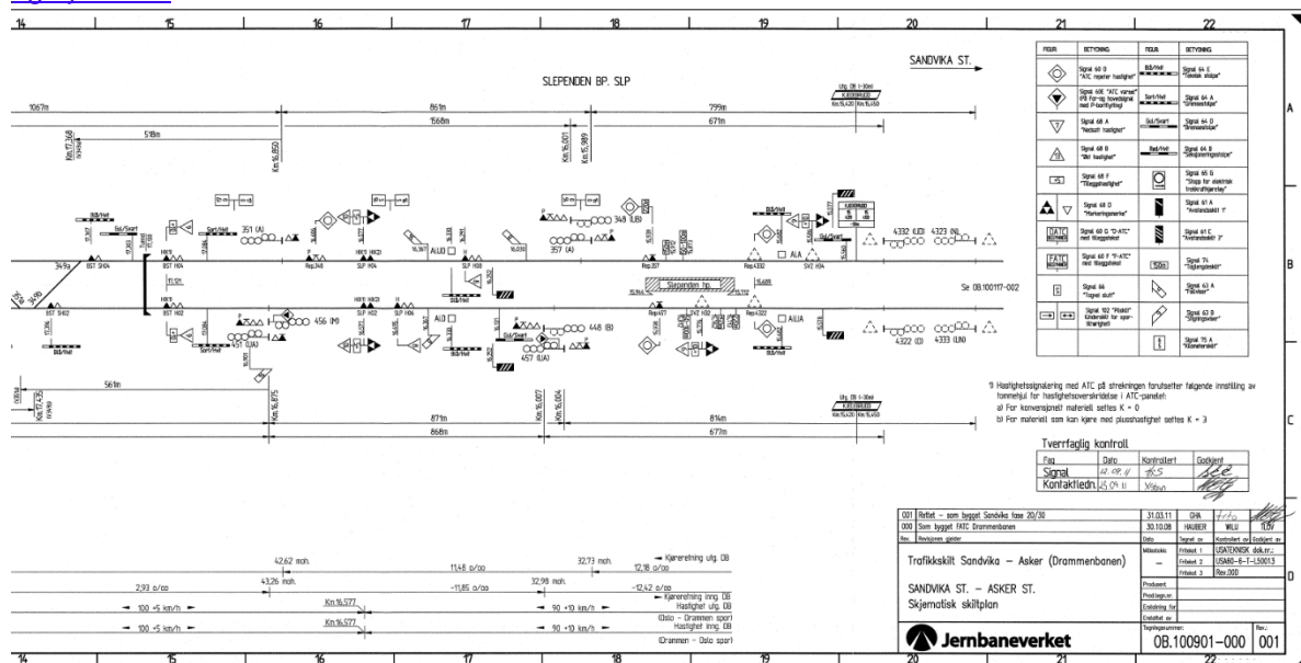
Figur 7: Eksempel på en skiltplan
