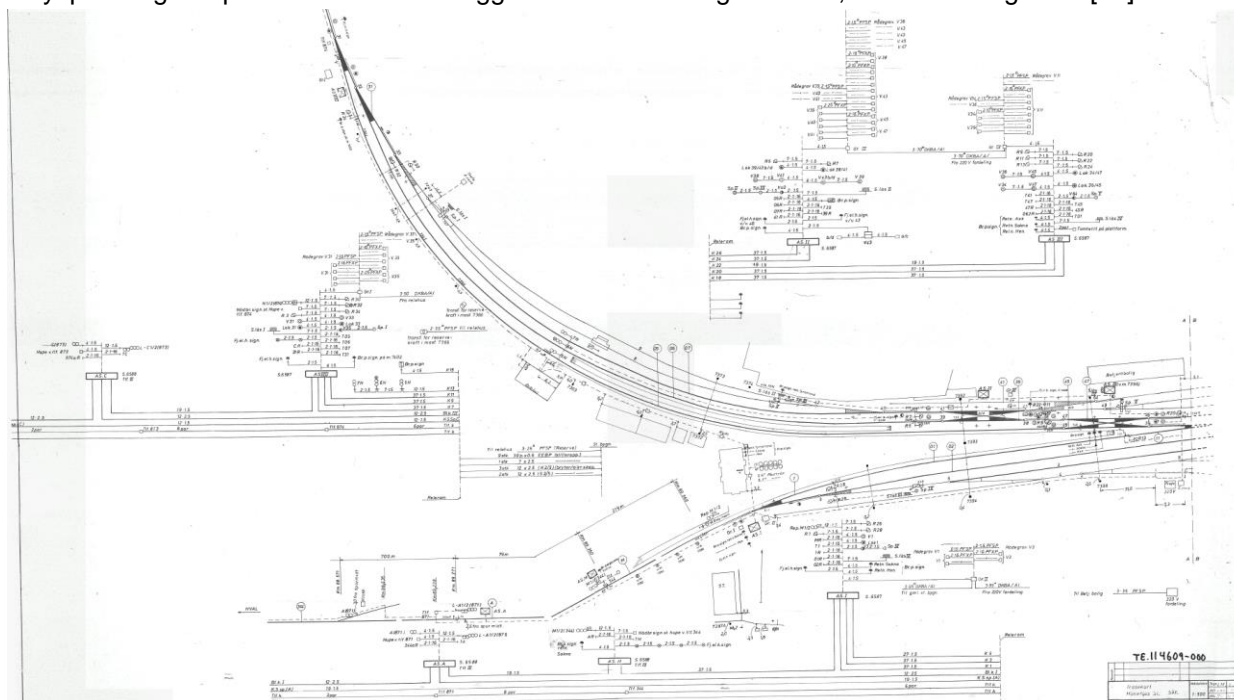
Figur 9: Eksempel på en kabeltrasekart.
